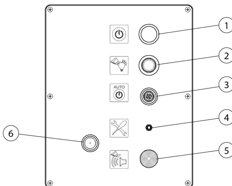
Fig 3: Elementos de mando
